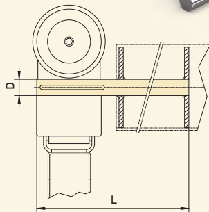
Aufsteck-ELEKTROMATEN SI + SIK mit Pendelfuß
