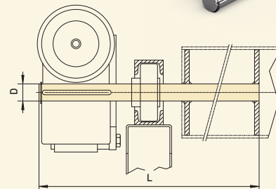
Aufsteck-ELEKTROMATEN SI + SIK mit Anroll-Drehmomentstütze
