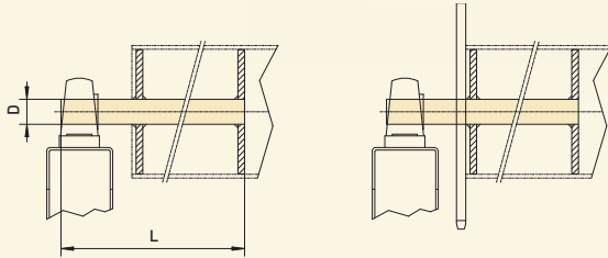
Lagerseite mit Kettenradscheibe
