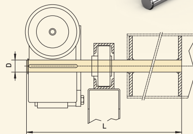
ELEKTROMATEN SI, SIK enchufables con apoyo de par para consola móvil
