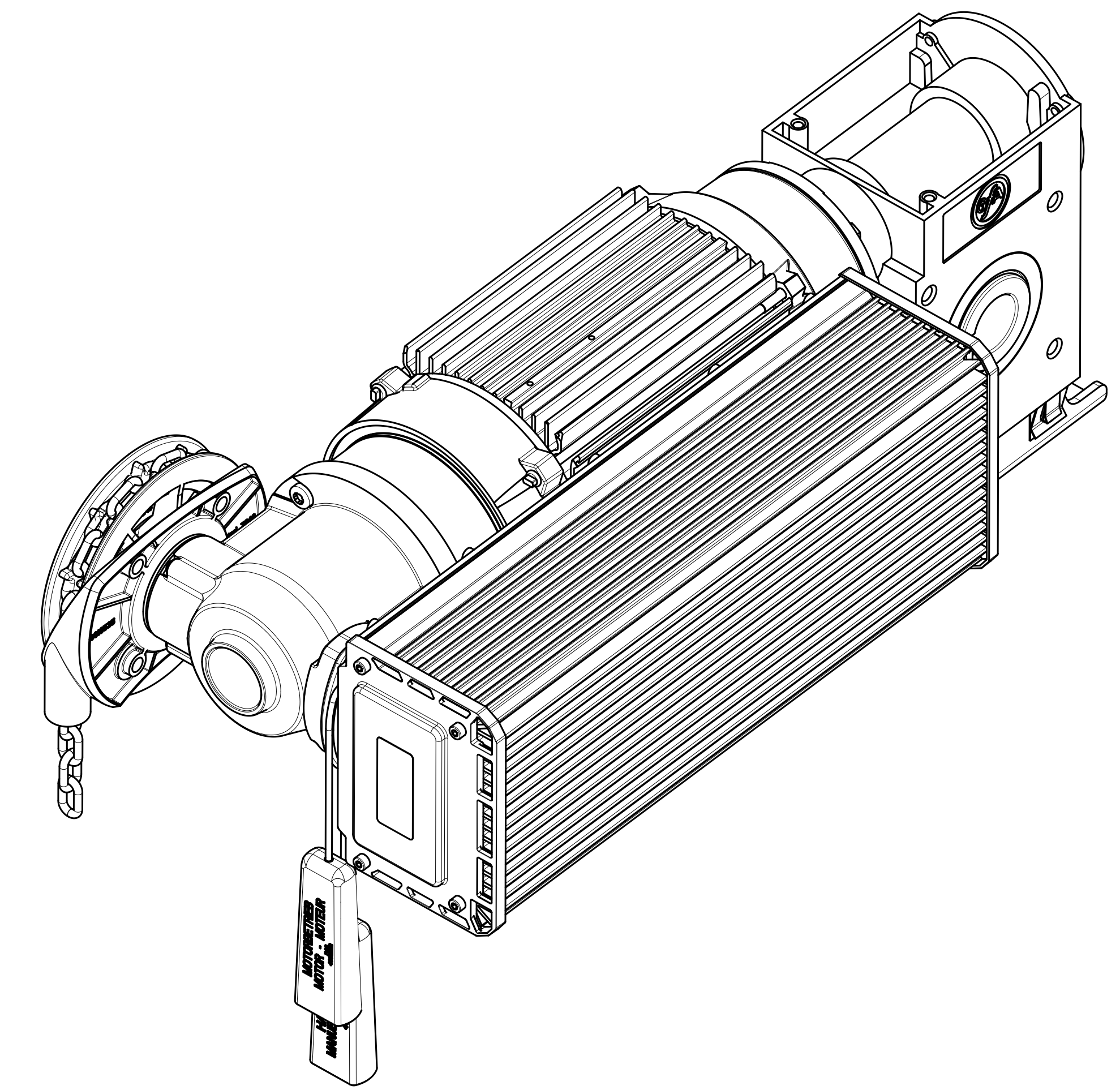
Darstellung: Einbaulage FU rechts illustration: FI on the right side
