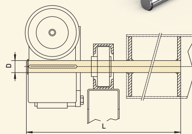
Motoréducteurs à prise directe ELEKTROMATEN SI, SIK avec flasque et doigt de maintien pour console à glissière
